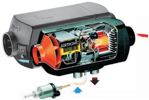
D2 Airtronic Cab Heater
